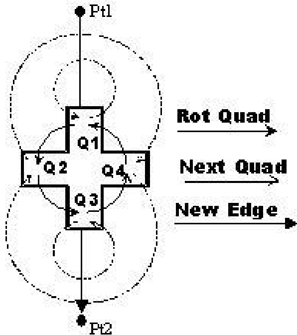
Figure 2.1 Make edge
